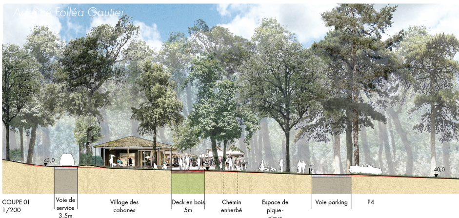
Coupe transversale de l'espace d'accueil
